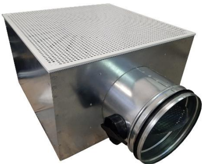
Perforált szögletes befúvó belső perdítő elemmel
